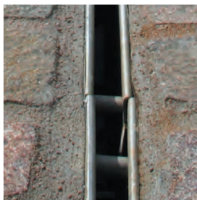
Aneinandergrenzende Schlitzrahmen ohne Connector Clip
